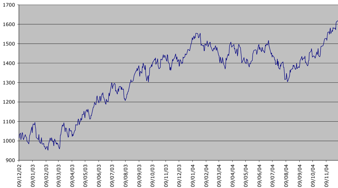
Nasdaq 100 indeksi
